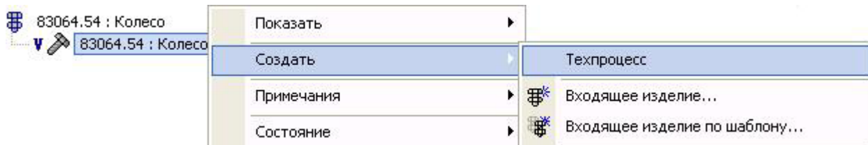
Рис. 3. Вызов модуля
