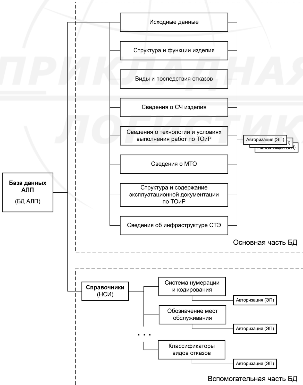
Рисунок А.1 — Логическая структура БД АЛП
