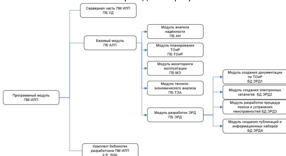
Рисунок 1. Взаимосвязь компонентов в составе ПМ ИЛП
